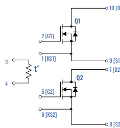
Dual MOSFET (4x6)
